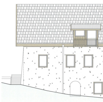
PROSPETTO SUD / OVEST
