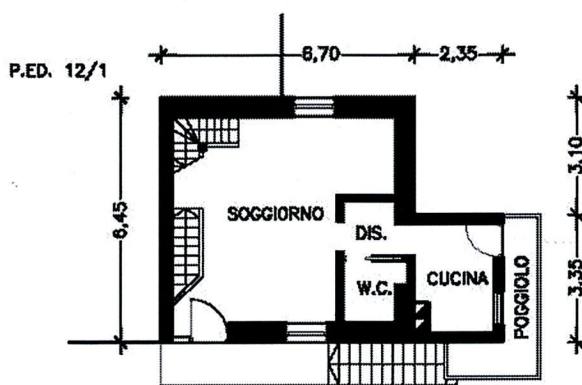
PIANO PRIMO H = m 2,40
