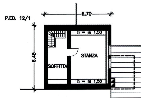
PIANO SECONDO H max = m 2,20 H min = m 1,25
